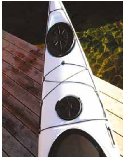
▲ Godt med luker av god kvalitet, men relativt tynt med strikk på dekk. Pluss for nedfelt kompassfeste
